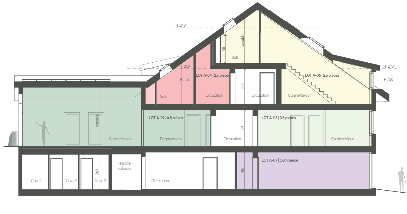
Coupe - 1/100 e
