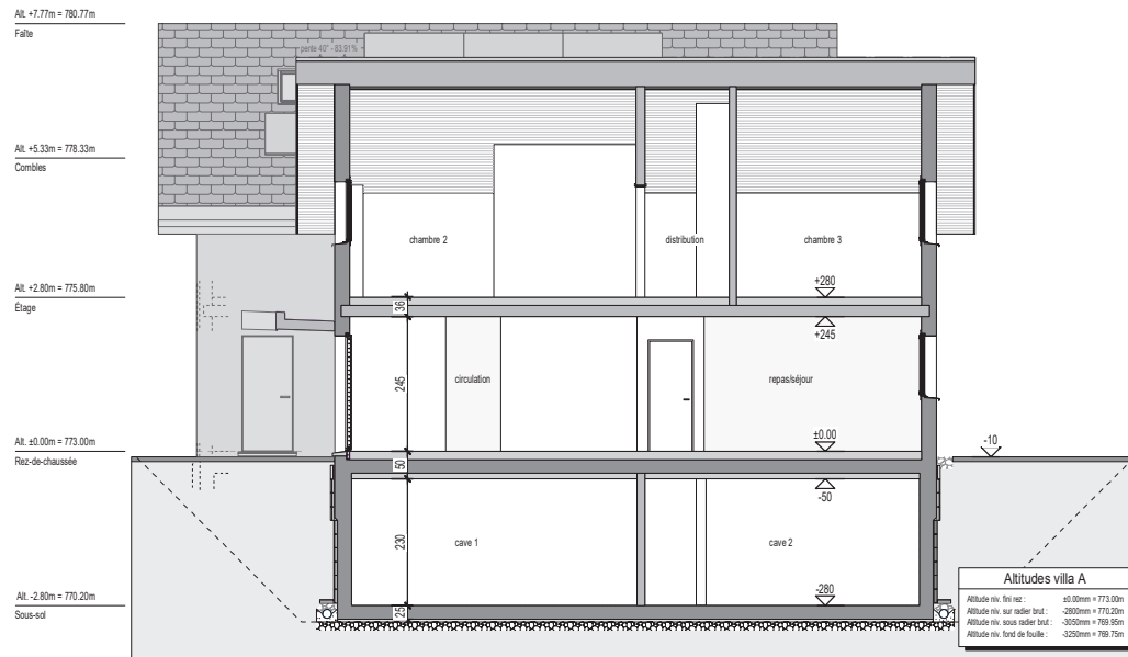
A-A Coupe - 1/100 e
