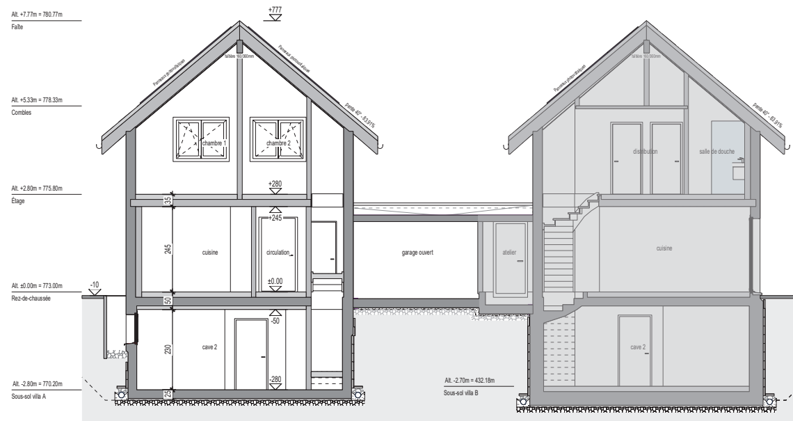
D-D Coupe - 1/100 e
