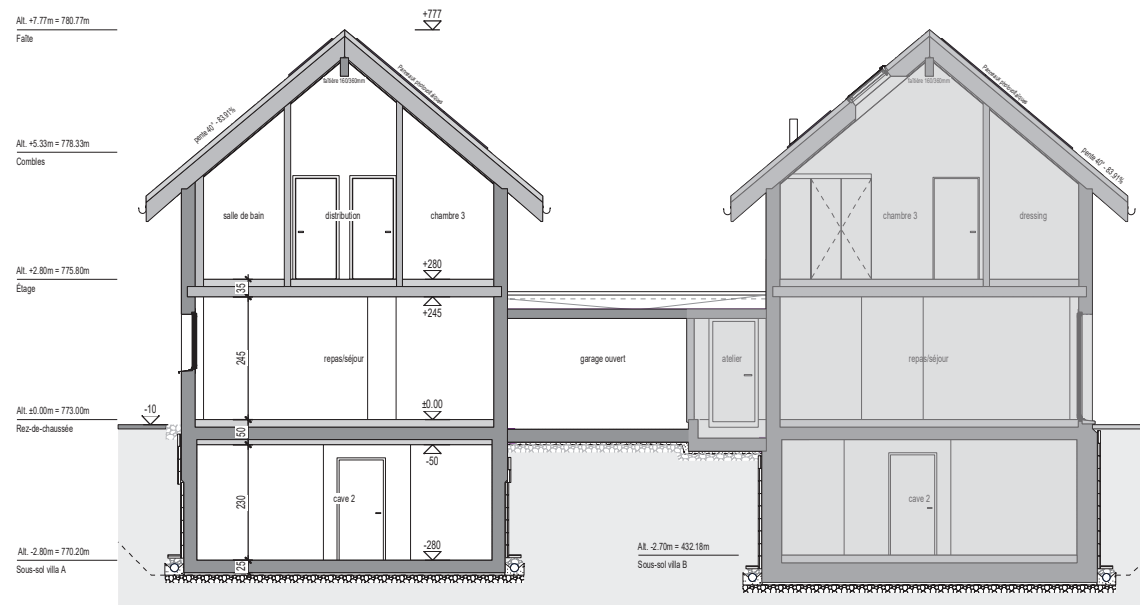
C-C Coupe - 1/100 e
