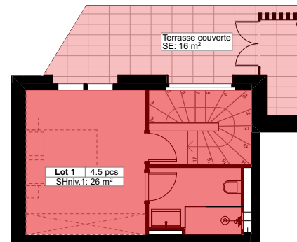
Niveau 1
